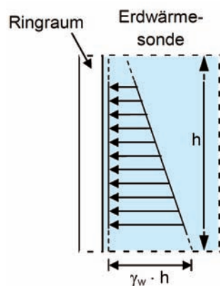
Abbildung 8: Erforderlicher Prüfdruck bei einem trockenen Bohrloch
