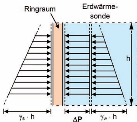
Abbildung 7: Erforderlicher Prüfdruck bei einem mit Bohrsuspension gefüllten Bohrloch
