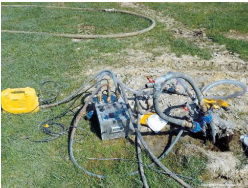
Abbildung 5: Dichtheitsprüfung der Erdwärmesonde [25]
