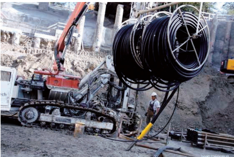
Abbildung 4: Haspel zum schonenden Einbau der Erdwärmesonde [25]
