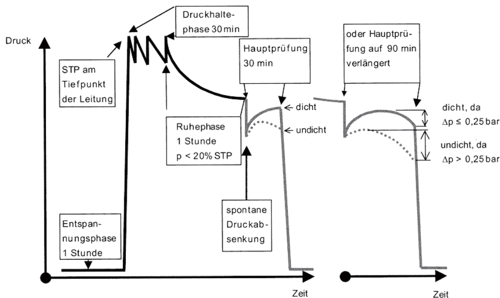
Abbildung 16: Beispiel für den Druckverlauf des Kontraktionsverfahrens bei einer dichten und einer undichten Druckleitung aus PE [8]
