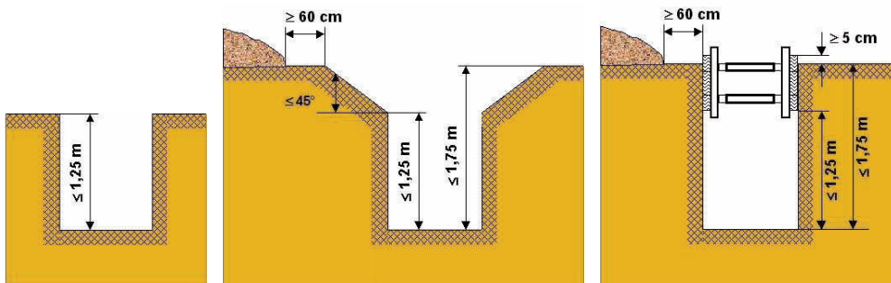
Abbildung 17: Sicherung von Rohrgräben gemäß DIN 4124 [10]
