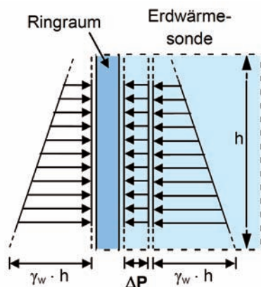
Abbildung 6: Erforderlicher Prüfdruck bei einem wassergefüllten Bohrloch
