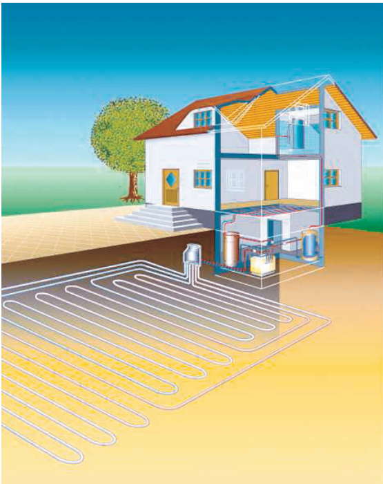
Abbildung 14: Systemskizze eines horizontalen Flächenkollektors [22]
