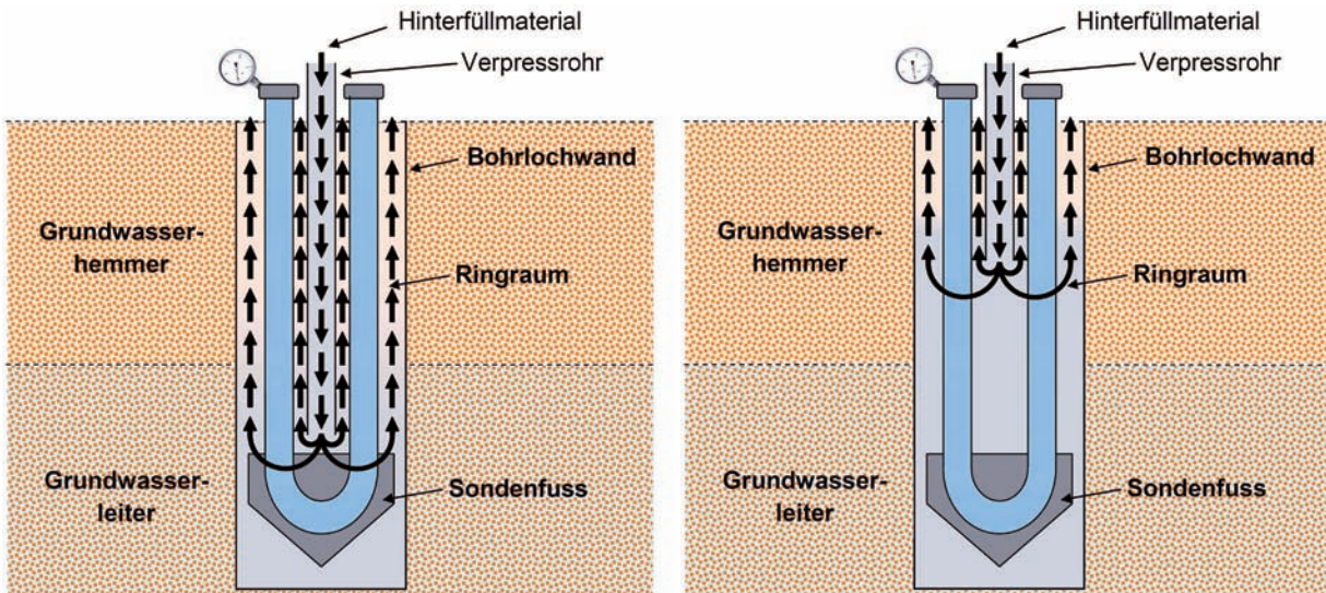
Abbildung 10: Verpressen des Hinterfüllmaterials mit kontinuierlichem Ziehen des Verpressrohres
